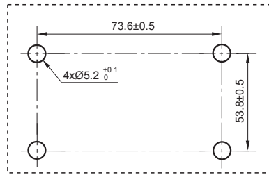
安装孔尺寸
