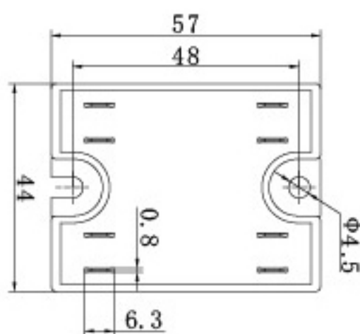
安装尺寸
