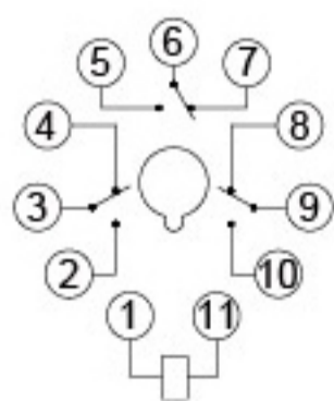
3Z接线图-2
