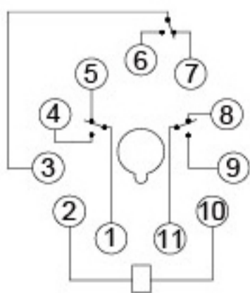
3Z接线图-1
