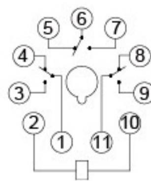
3Z接线图-3
