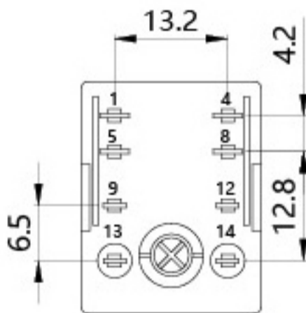
安装尺寸
