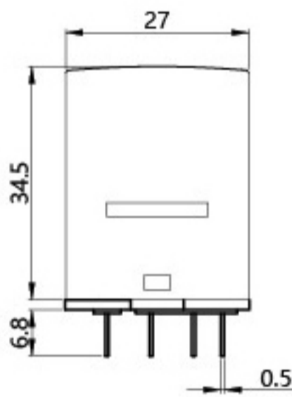
正面图
