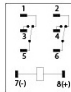
接线图
